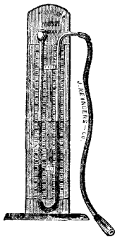
Fig. 312. Pneumatometer.
